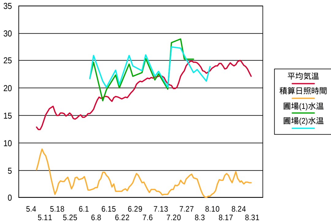
図3 アメダス角館の平均気温と水田水温 (午前 9時 )の推移 1995年度 過去 7 日間の移動平均
