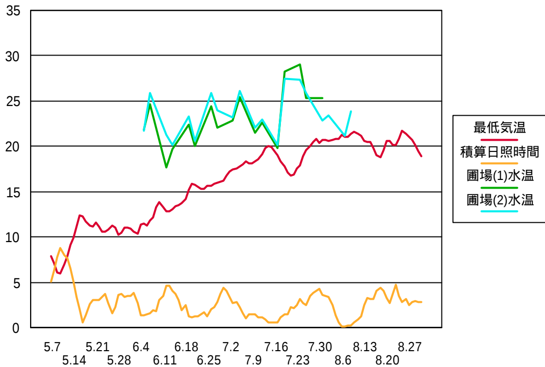
図2 アメダス角館の最低気温と水田水温 (午前 9時 )の推移 1995年度 過去 7日間の移動平均
