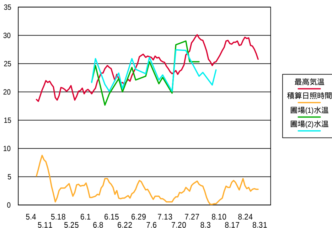
図１ アメダス角館の最高気温と水田水温 (午前９時)の推移 １９９５年度 過去７日間の移動平均
