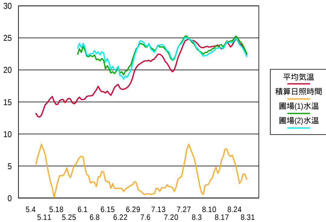
図3 アメダス尾花沢の平均気温と水田水温 (午前 9時 )の推移 1995年度 過去 7 日間の移動平均
