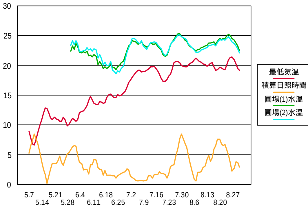
図2 アメダス尾花沢の最低気温と水田水温 (午前9時)の推移 1995年度 過去7日間の移動平均
