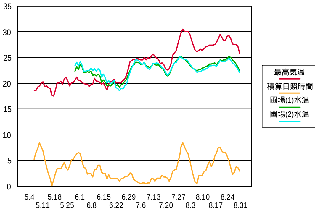
図１ アメダス尾花沢の最高気温と水田水温（午前９時）の推移 １９９５年度 過去７日間の移動平均
